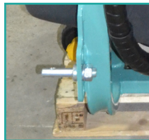
Kačenje u tri tačke Three point coupling
