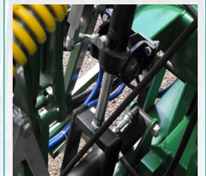
Hidraulična korekcija grana Hydraulic leveling booms
