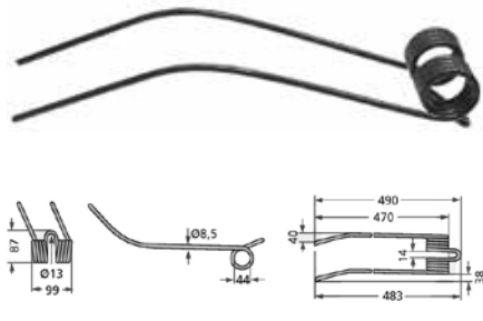
Opruga sakupljača Kuhn: GA 230, 280, 300
