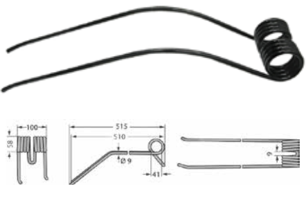
Opruga sakupljača Kuhn: GA 230, 280, 300, 301, 402, 3201
