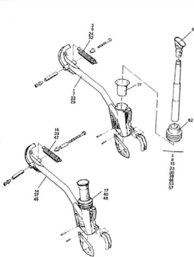
Teleskopska cijev metalna, duža, univerzalna
