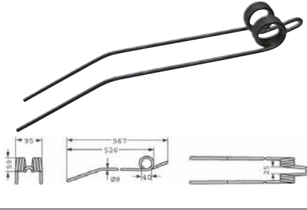
Opruga sakupljača Deutz Fahr: KS 83, 85, 90, 200, 300
