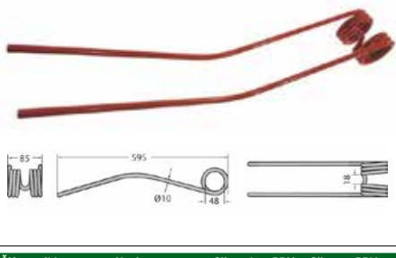
Opruga sakupljača Claas: Liner 390, 430, 470, 650, 680, 780, 880, 1550, 3000
