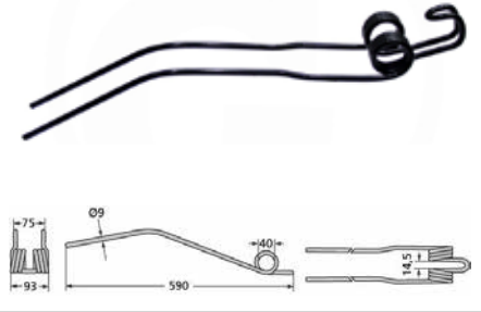
Opruga sakupljača Deutz Fahr: KS 1.70, 2.33, 2.37, 2.60
