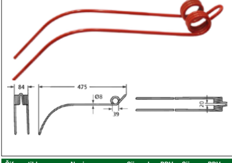
Opruga sakupljača Claas: WS 280, 310 PZ: Andex 280, 310, 330
