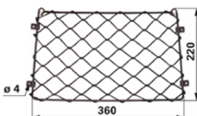
Mreža stražnjeg zida traktora 360 x 220 mm
