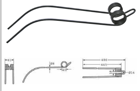
Opruga sakupljača Deutz Fahr: KS 6, 8, 60, 80
