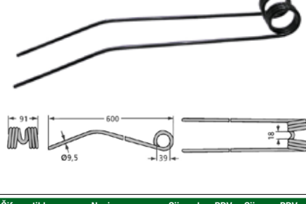
Opruga sakupljača Fella: TS 290, 295, 320, 330, 335, 415, 630, 631
