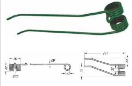
Opruga sakupljača Fella: TS 7, 8, Fum 320 Stoll: UM 320, 321, 410
