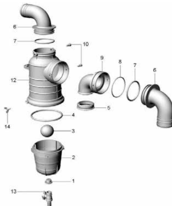
Kugla PVC 80 mm
