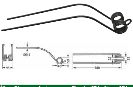
Opruga sakupljača Fella: TS 425, 455, 781, 1600
