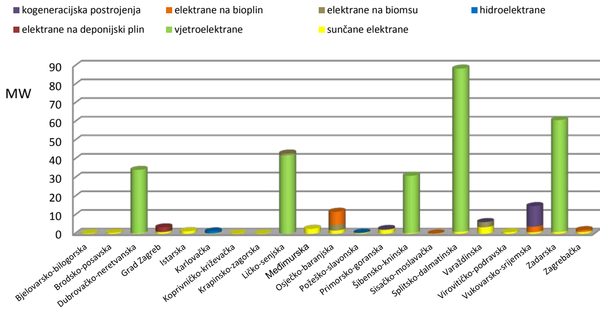
Slika 11: Prikaz ukupne instalirane snage po županijama
