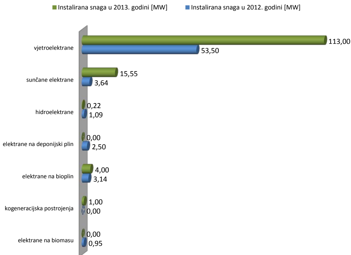
Slika 10. Prikaz instalirane snage elektrana koje su ušle u trajni pogon u 2012. i 2013. godini
