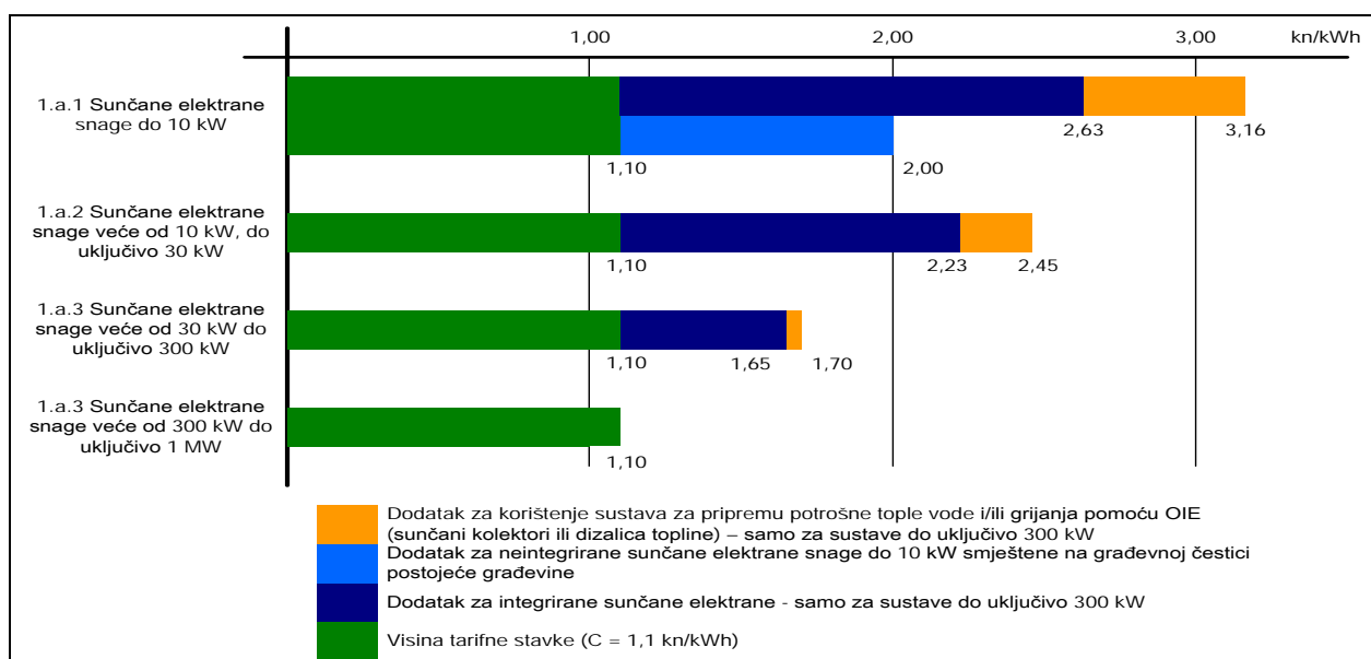
Slika 3. Tarifni sustav za integrirane sunčane elektrane
