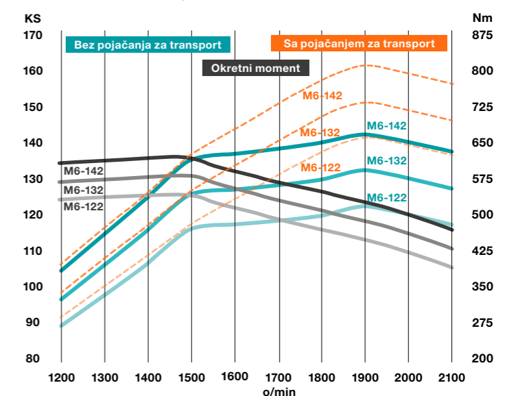
Okretni moment, snaga motora sa i bez pojačanja za transport
