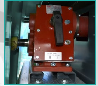
Reduktor sa dve brzine Gearbox with two gears
