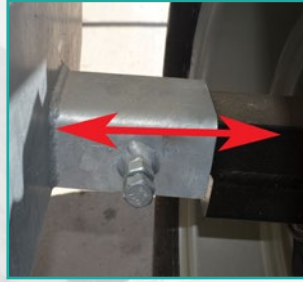
Osovina podesiva po širini i visini Width and height adjustable axle
